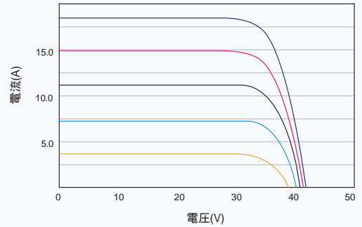
PVモジュール (600W) P-V 曲線
